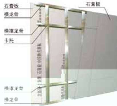
无贯通龙骨隔墙示意图
